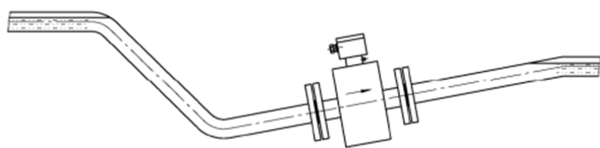
Рис. 4 Монтаж в заполненных трубопроводах
