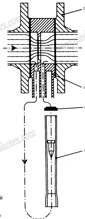
а Датчик дифференциального давления с измерительной диафрагмой b Фланец трубопровода c Поплавковый расходомер d Байпасная диафрагма
